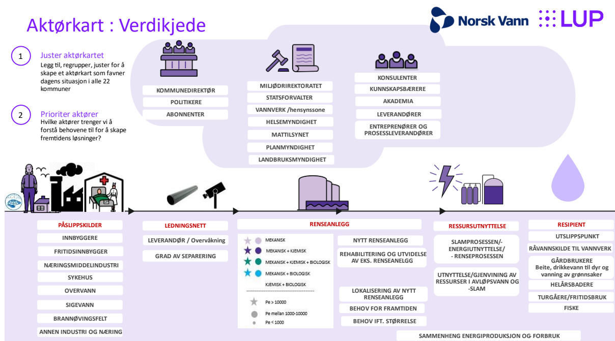
Figur 3: Aktørkart / verdikjede
